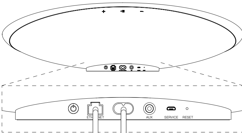
図3 有線設定接続
