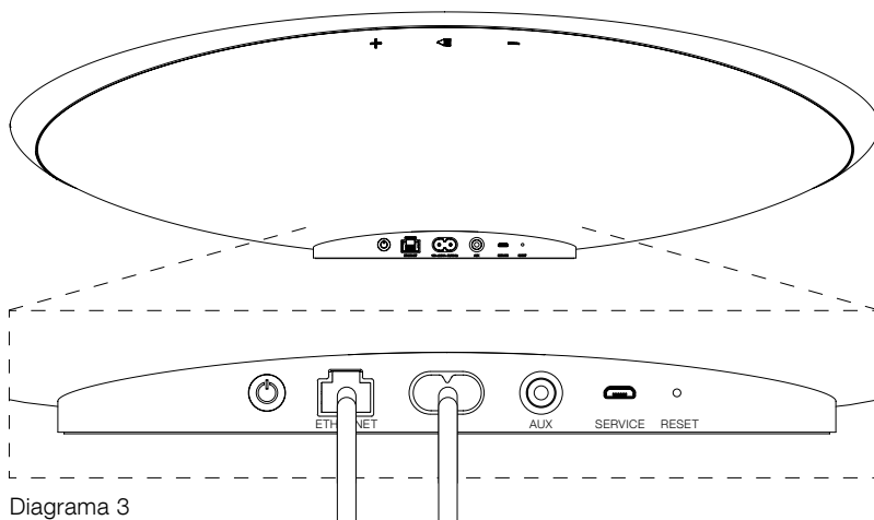
Diagrama 3 Conexión para configuración por cable
