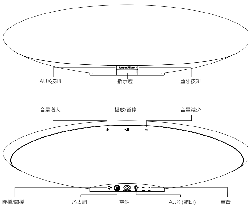
圖1 按鈕和連接插孔
