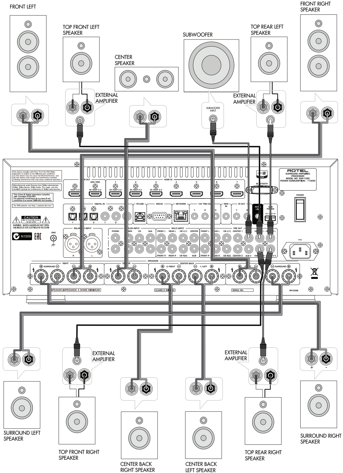
Luidspreker verbindig Collegamento degli altoparlanti Högtalaranslutning Подключение громкоговорителя
